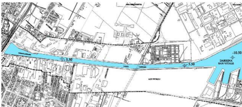
Figura 33 - Planimetria Porto di Ravenna 3/3 (Darsena di Città) - Fonte: PRP – AdSP
